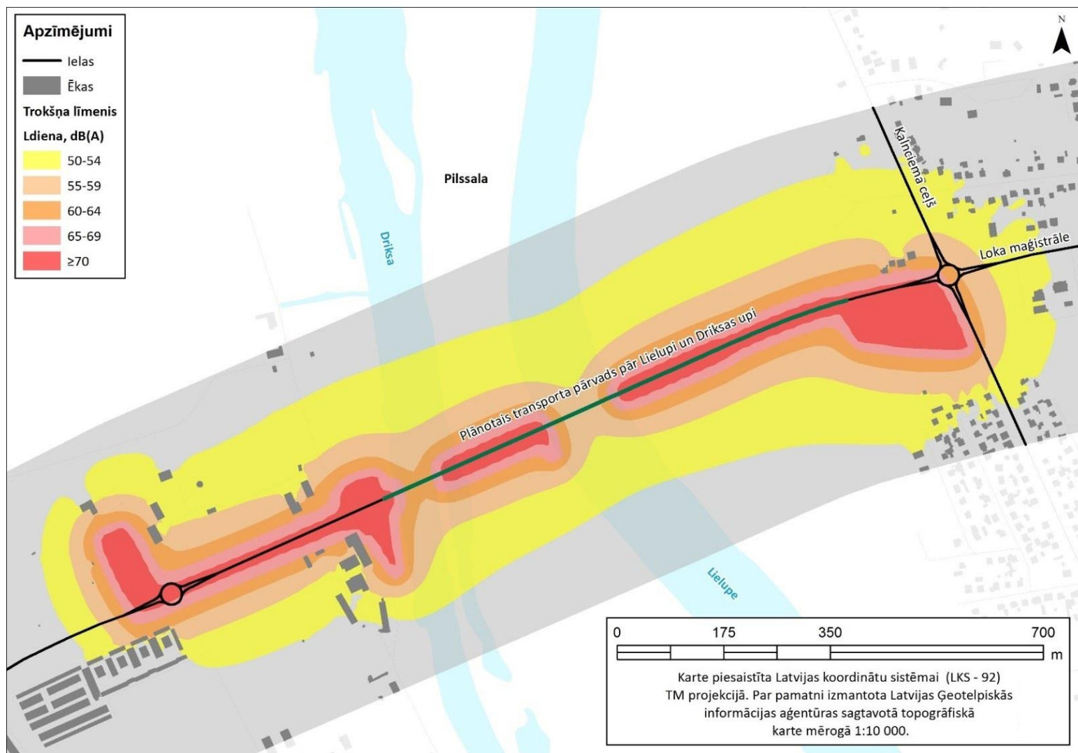
Aprēķinātais trokšņa līmenis transporta pārvada būvniecības laikā trokšņa rādītājam L_{diena}
