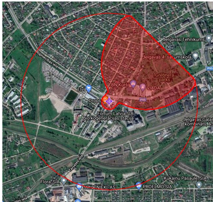
24. attēls. Benzīnaoplūdes no DUS toksisko tvaiku izplatība
