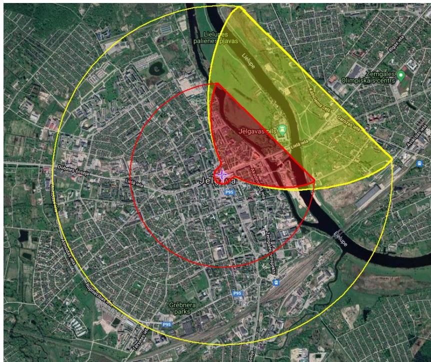
45. attēls. Tvaika mākoņa uzliesmošanas zona
