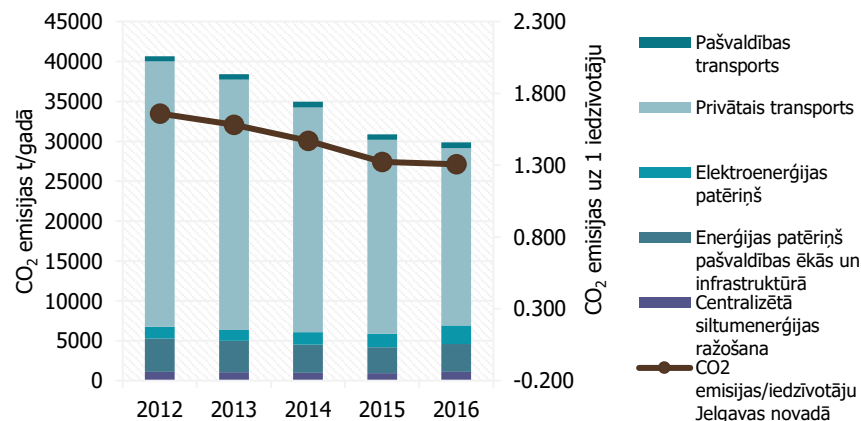
Attēls 14.1.1. CO 2 emisiju apjoms bijušā Jelgavas novadā 2012.–2016. gadā
